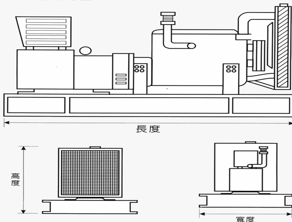
柴油發電機組尺寸圖
